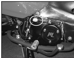
Tapa del orificio de llenado del aceite y bayoneta de nivel de aceite.
